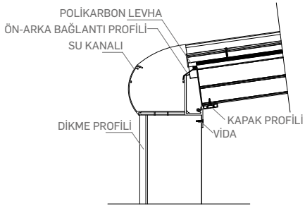
Dikme & Ara Bağlantı & Su Kanalı Detayı
