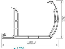
• 1791 Oluk Profili BORDER PROFILE Ağırlık / Weight: 5,742
