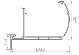
• 1656 Oluk Profili BORDER PROFILE Ağırlık / Weight: 4,046
