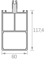
• 1653 Griyaj Profili GRIYAJ PROFILE Ağırlık / Weight: 2,724
