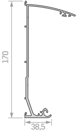
• 1658 Duvar Sabitleme Profili WALL FIXING PROFILE Ağırlık / Weight: 2,086
