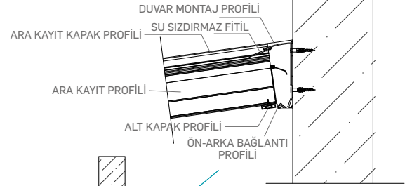
Duvar Bağlantı Detayı
