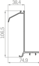
• 5707 Geçme Açı Profili ANGLE PROFILE Ağırlık / Weight: 1,073
